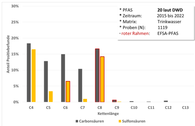
Abb. 3: Häufigkeitsverteilung der PFAS nach Kettenlänge in deutschen Trinkwässern
