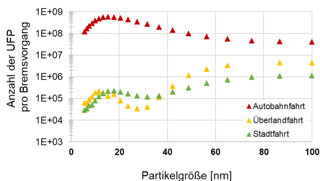
Abb. 5: Partikelanzahl und Größenverteilung der emittierten UFP (6-100 nm, HR-ELPI+)
