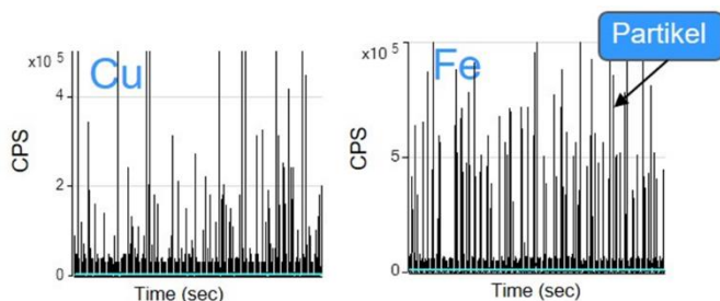
Abb. 3: Beispielspektren von ultrafeinen Metallen (SP-ICP-MS)
